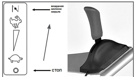
Рис. 12 Положение рычага газа при запуске двигателя
