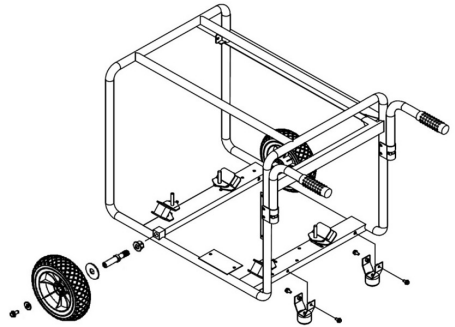
Рис. 4 Установка транспортировочных колес и опор рамы
